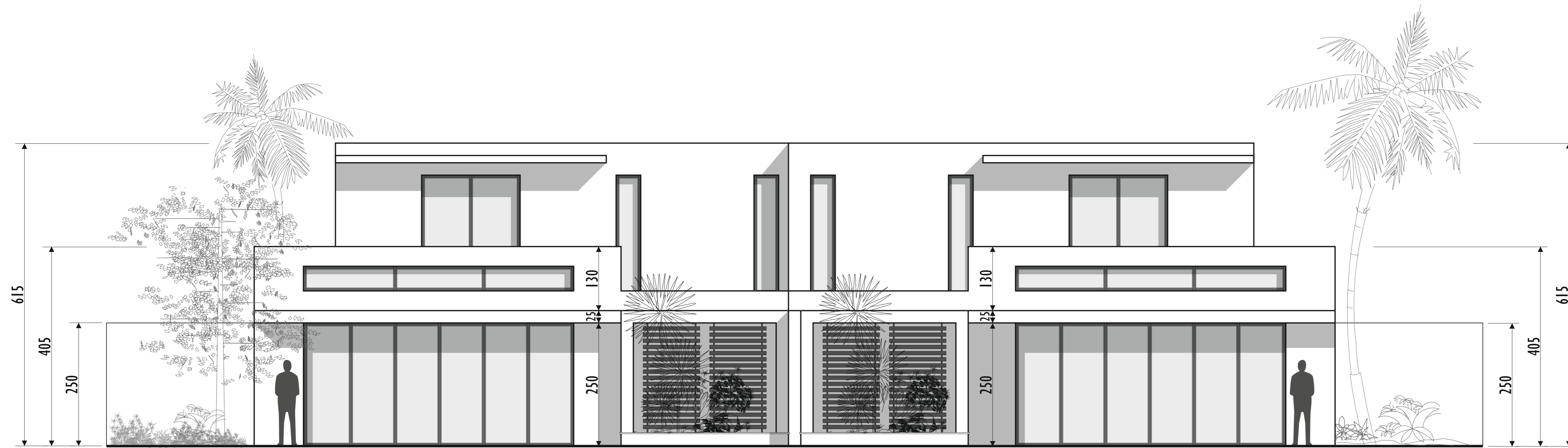
ELEVACION SUR
